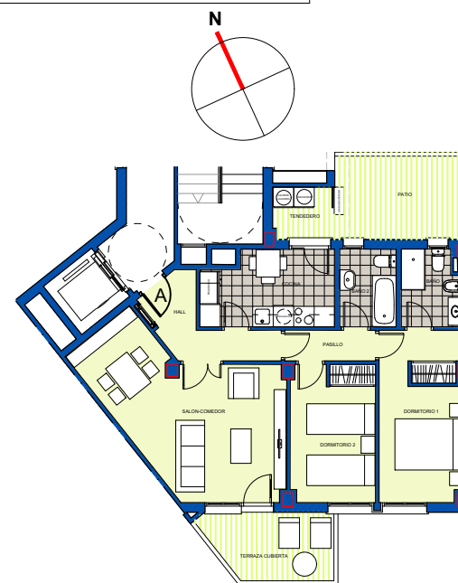
ESCALA: 1 / 200
