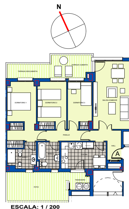
ESCALA: 1 / 200
