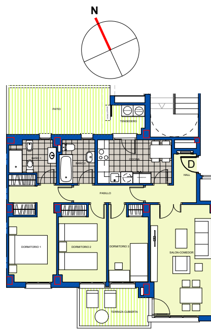
ESCALA: 1 / 200
